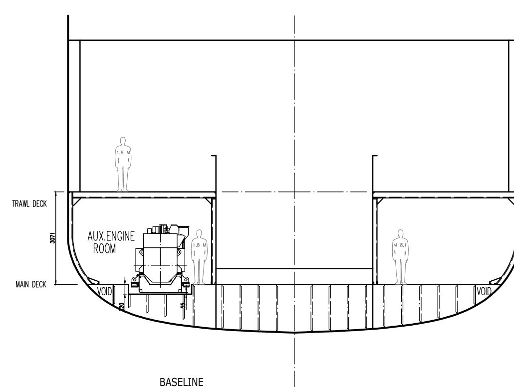
FRAME -3
