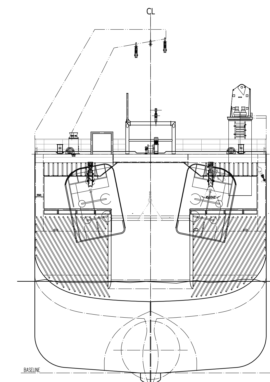
TRANSOM
