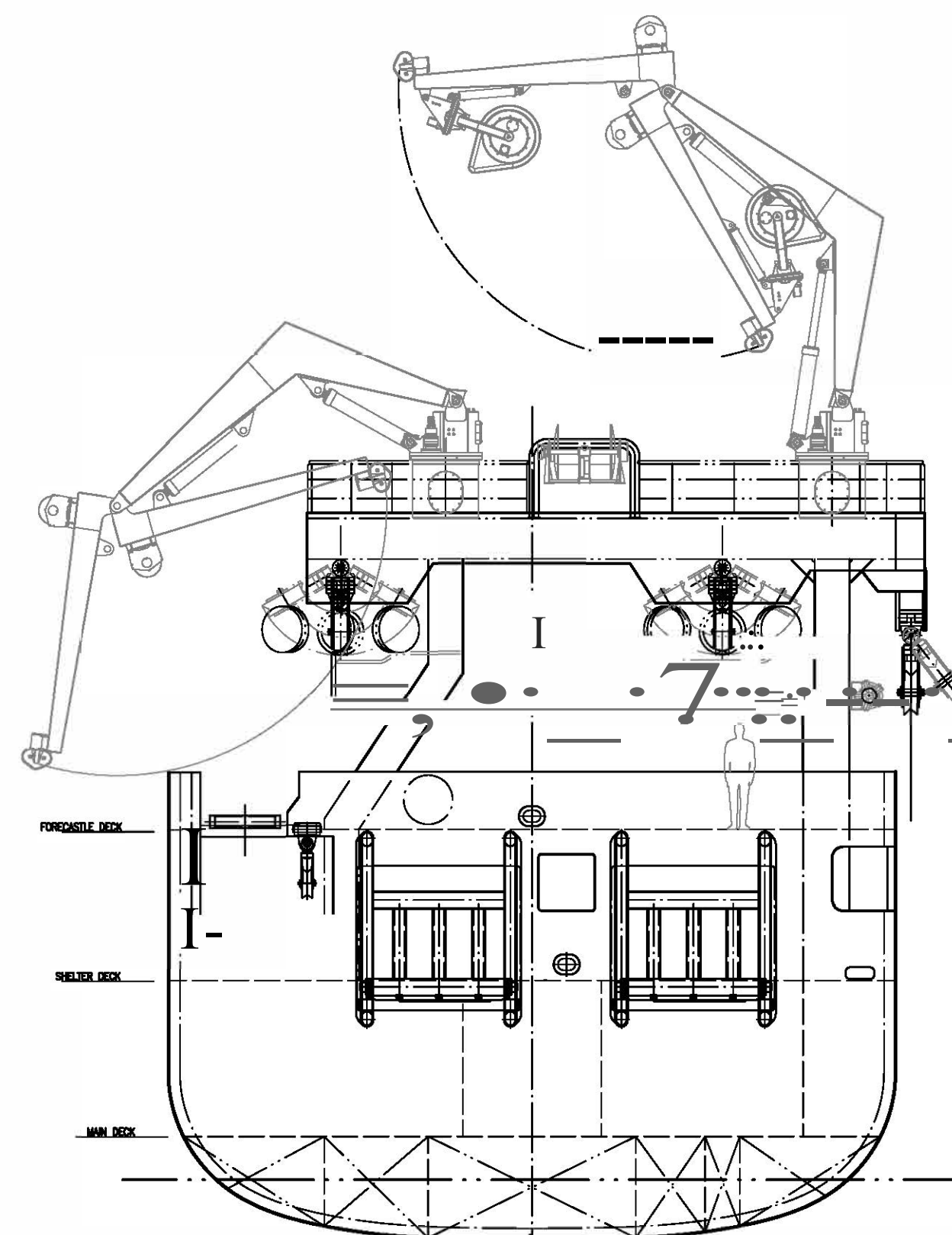
9L FRONTVIEW
